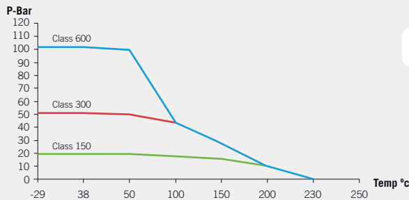
Fig. 2515 (Class 150)
