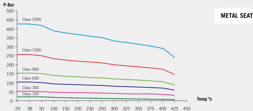
Fig. 6015 (Class 150)
