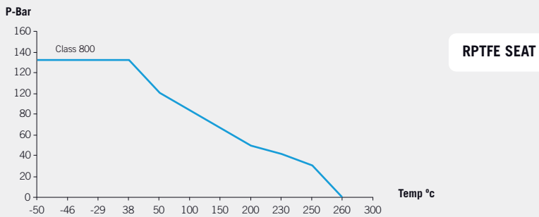
Fig. 400 (Class 800)
