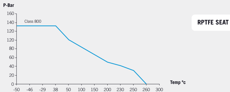
Fig. 800 (Class 800)
