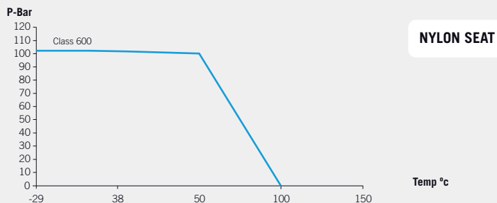
Fig. 560 (Class 600)
