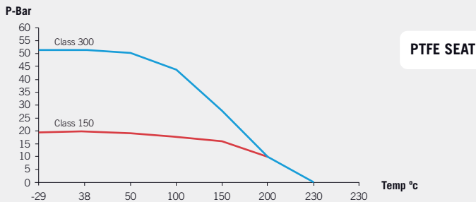
Fig. 1515 (Class 150)
